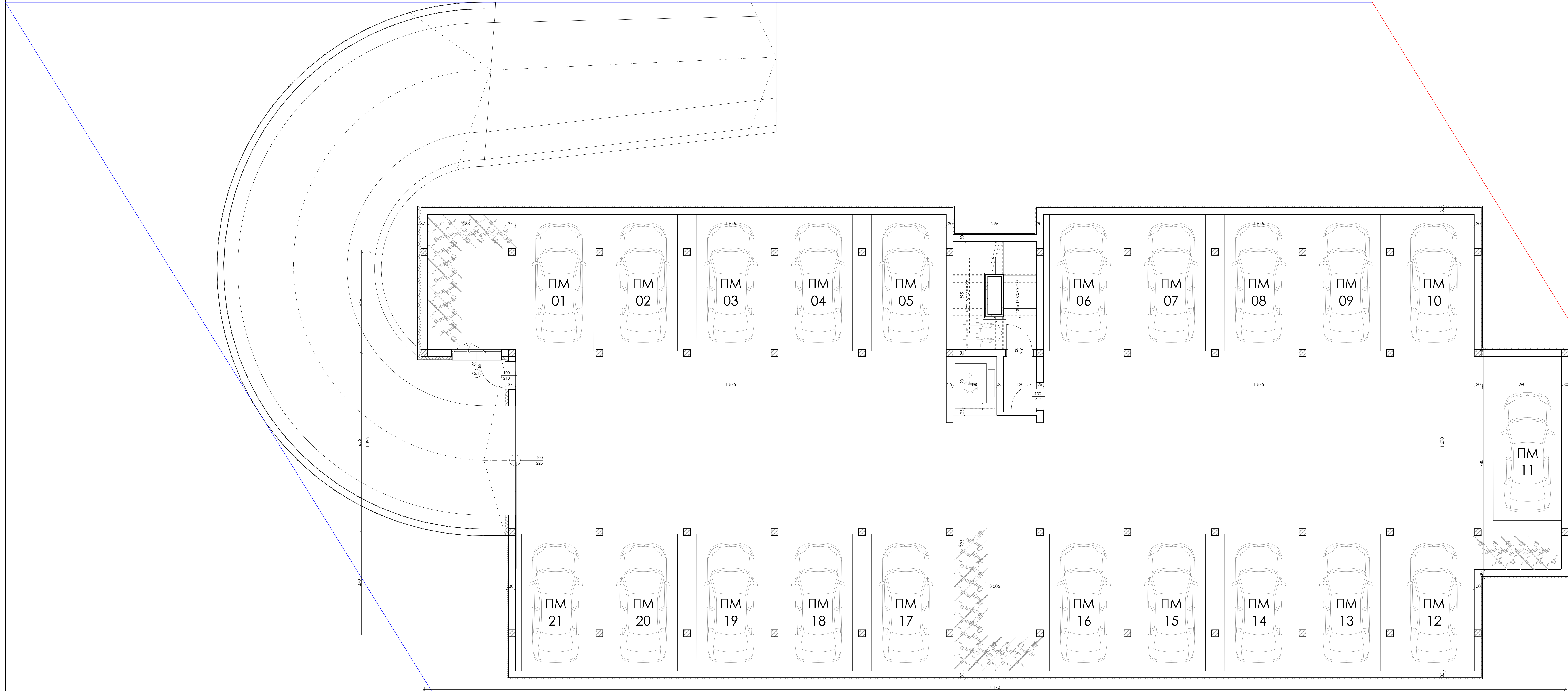
КОТА -2.85 ЕТАЖ -1 /СУТЕРЕН/
