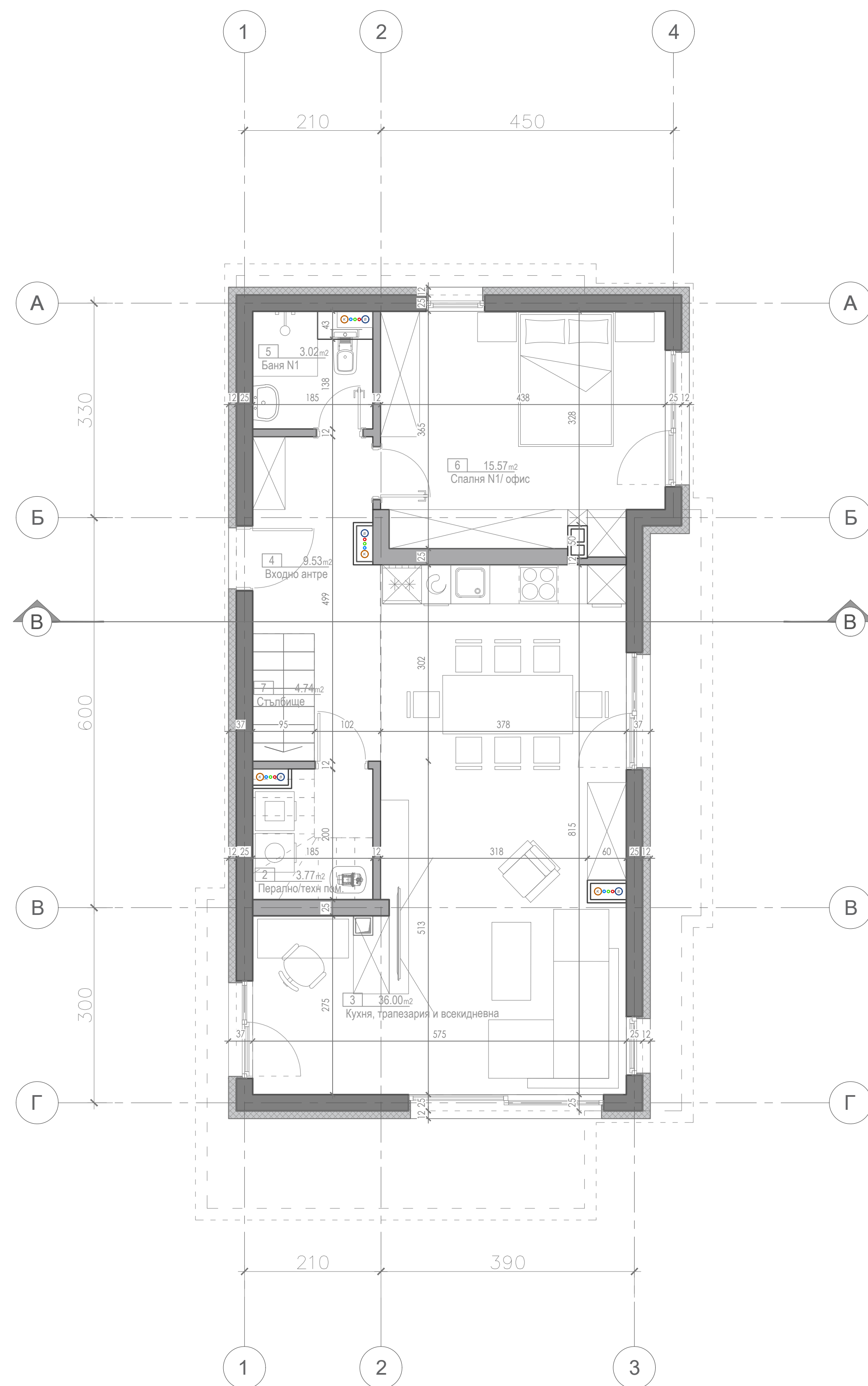
Къща В — ет.1 80,56 м² РАЗПРЕДЕЛЕНИЕ КОТА ±0.00
