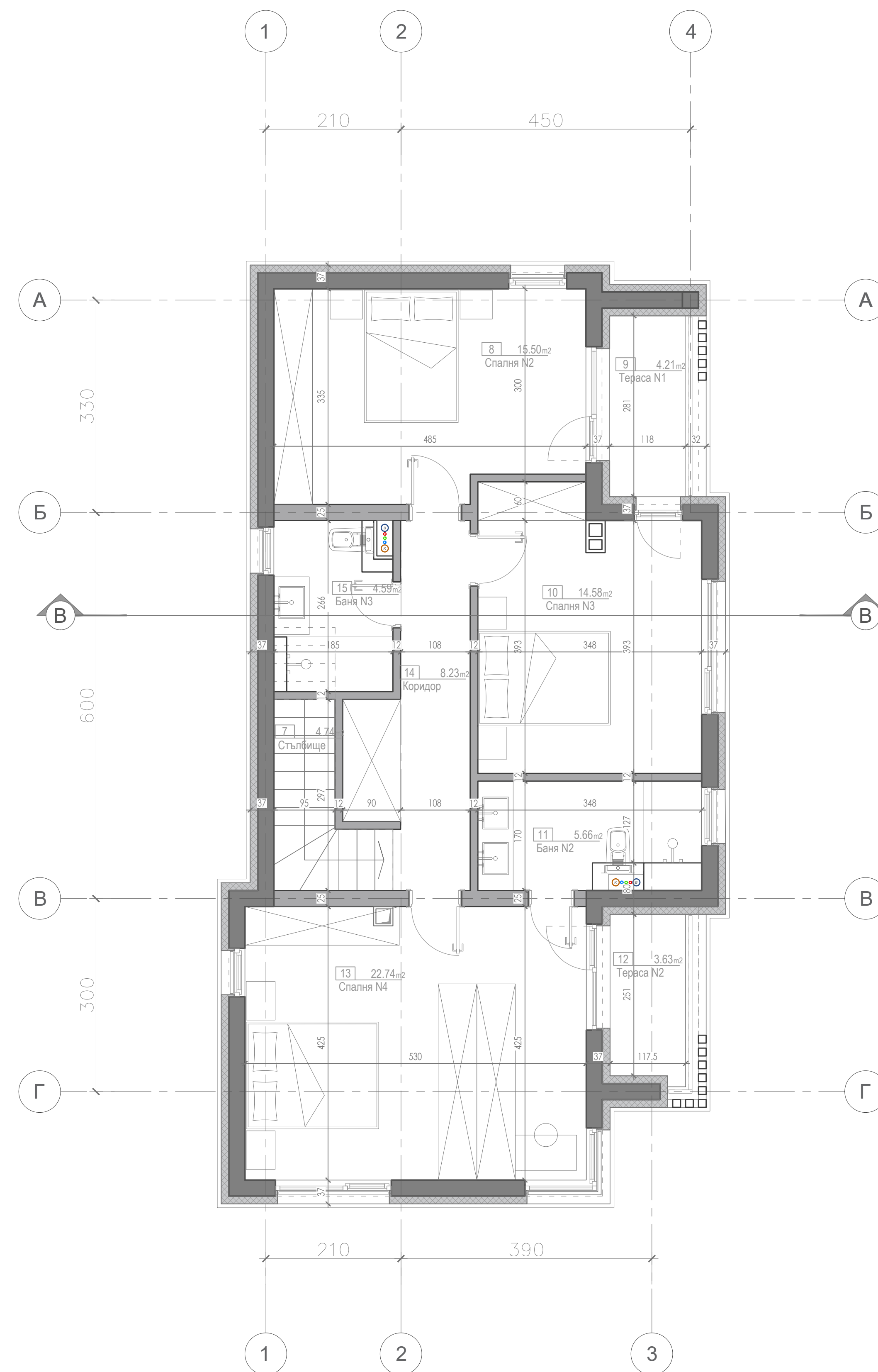
Къща В — ет.2 99,62 м² РАЗПРЕДЕЛЕНИЕ КОТА +3.10
