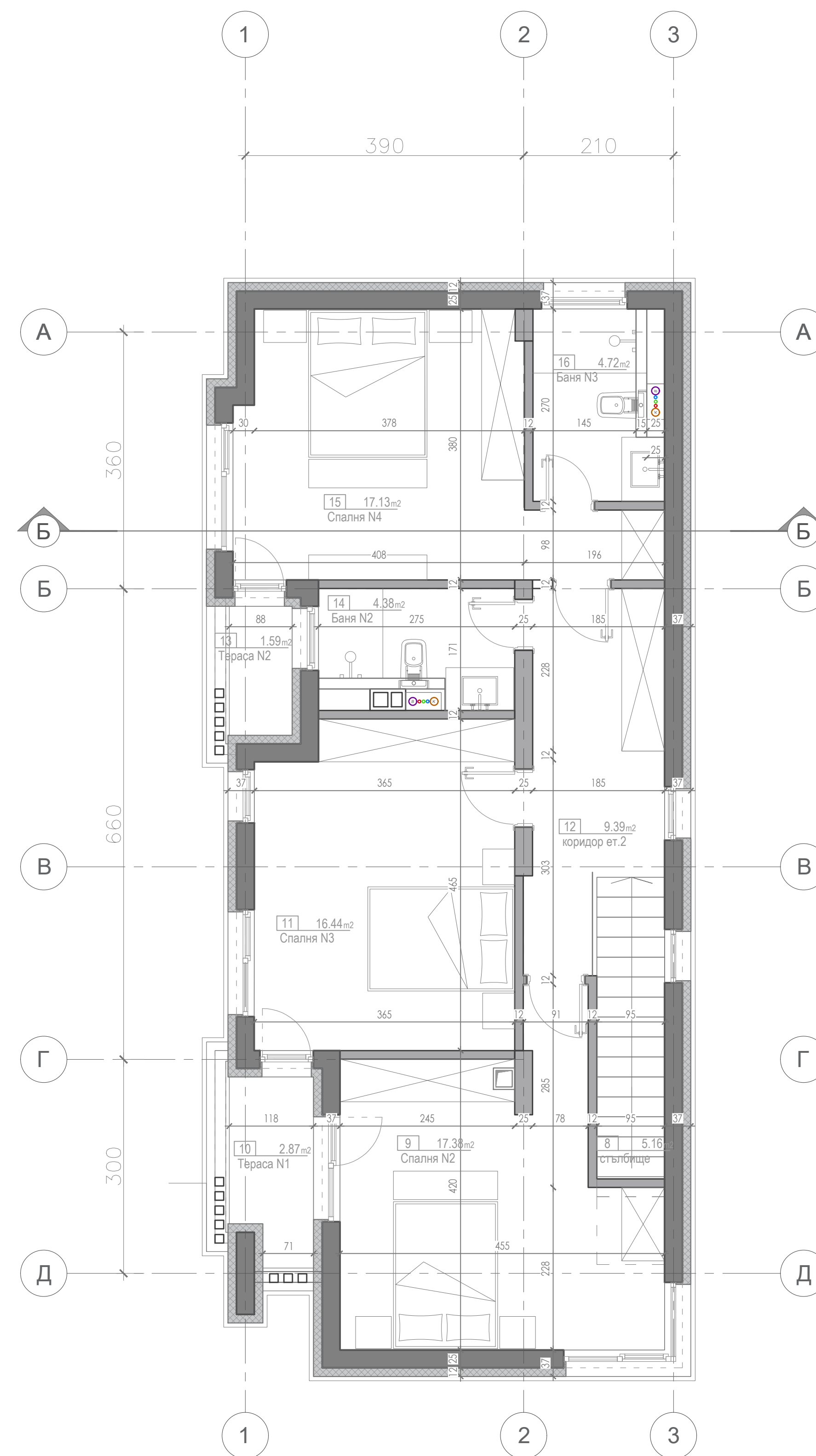
Къща Б — ет.2 95,40м 2 РАЗПРЕДЕЛЕНИЕ КОТА +3.10
