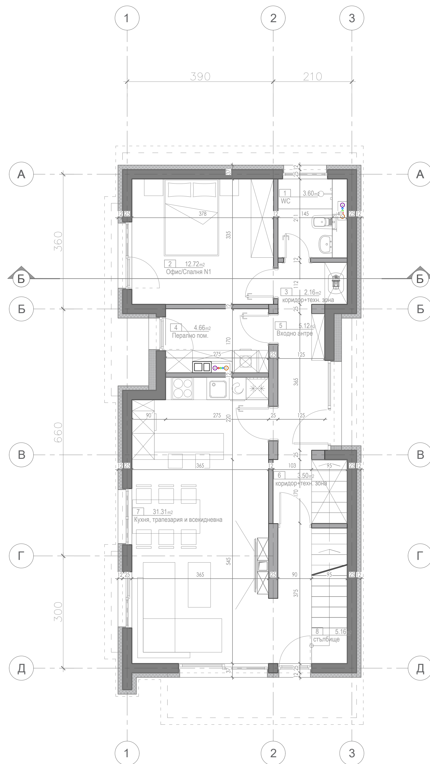
Къща Б — ет.1 80,14м 2 РАЗПРЕДЕЛЕНИЕ КОТА ±0.00
